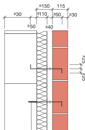
HMOŽDINKA DO BETONU, PLNÉ CIHLY A POROBETONU
