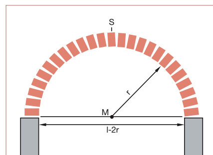
Kruhový oblouk
