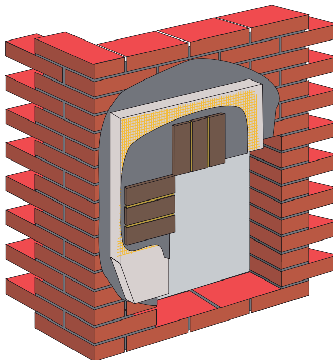
Obklad v místě stavebního otvoru
