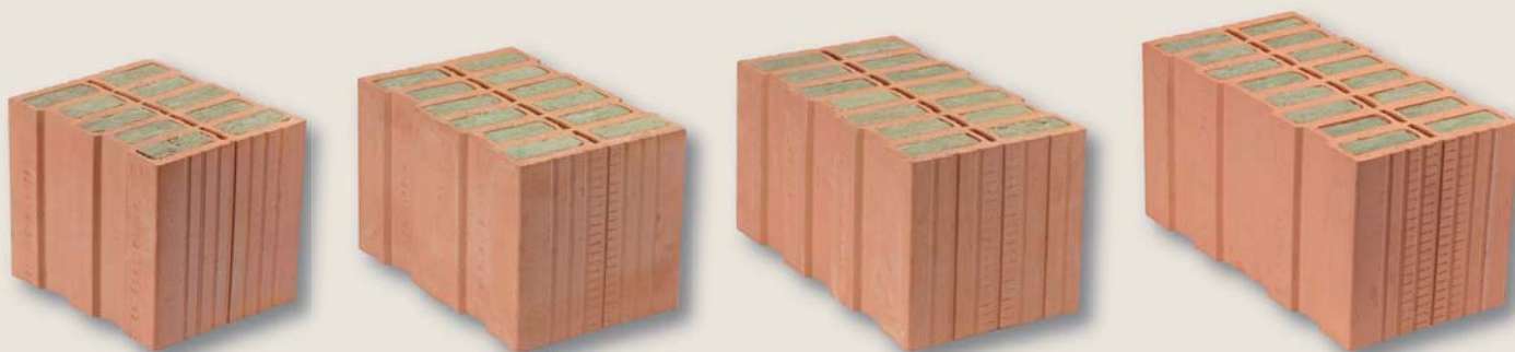
Dvojblok polovičních cihel Porotherm 30 T Profi 1/2
