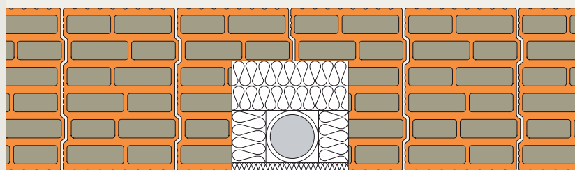
7.12.2 Druhá vrstva cihel Porotherm 38 T Profi u vyzdívané drážky pro odpadní potrubí.
