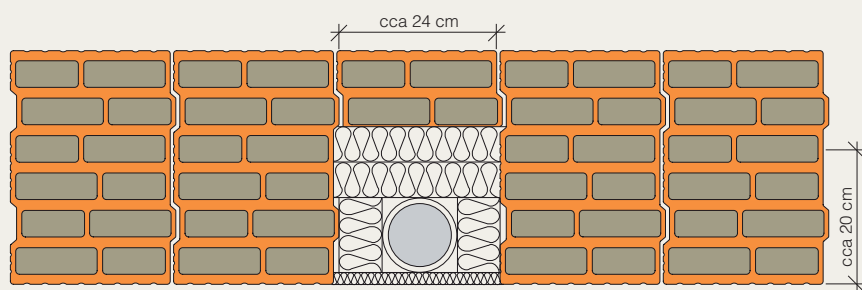
7.12.1 První vrstva cihel Porotherm 38 T Profi u vyzdívané drážky pro odpadní potrubí.
